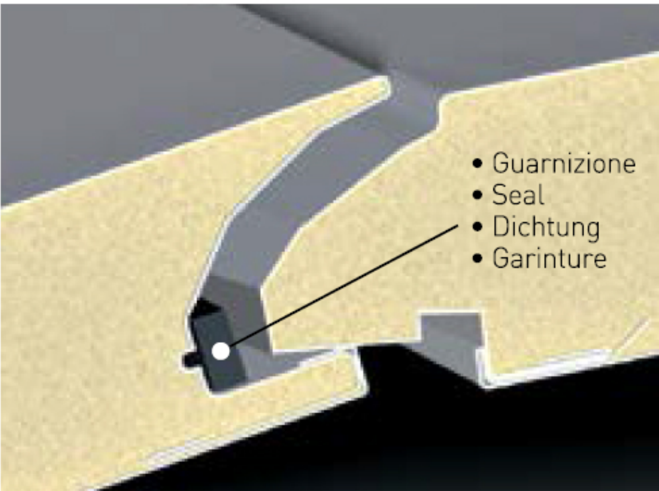
Particolare dell'accoppiamento Detail of joint Detail der Verbindung Détail du joint
